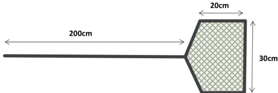
Figuur 2.4 Standaard macrofaunahandnet (conform NEN-EN-ISO 10870:2010)
