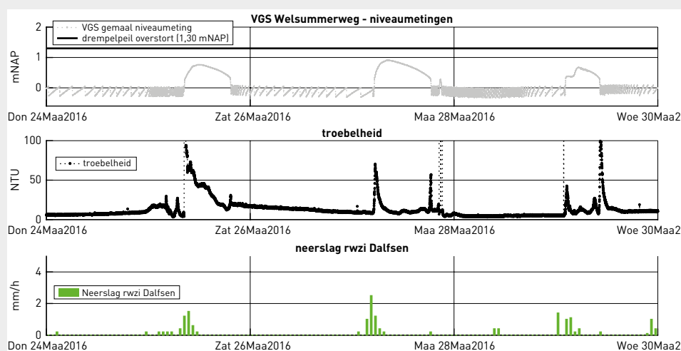
Figuur 6.5 Voorbeelden 'first flush' en 'final flush' uit praktijkproef Dalfsen: pieken in troebelheid (middelste grafiek) bij aanvang van de neerslag (onderste grafiek) en als het stelsel weer bijna is leeggepompt (bovenste grafiek)
