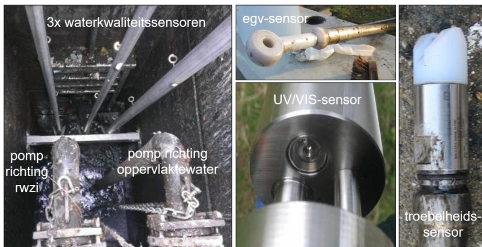
Figuur 6.3 Waterkwaliteits-sensoren toegepast in VGS 2.0-hemelwatergemaal
