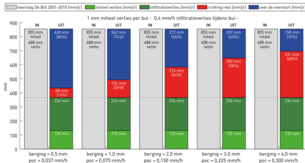
Figuur 4.4 Gevoeligheid jaarbalans en verdeling over afvoerroutes voor grootte berging en pompovercapaciteit, bij gelijkblijvende ledigingstijd van 13,3 uur
