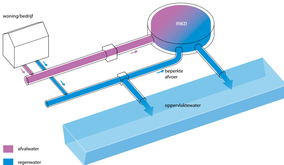
Figuur 2.1 Principeschema verbeterd gescheiden rioolstelsel (Bron: Riolerings in Beeld, Benchmark Rioleringszorg 2013)
